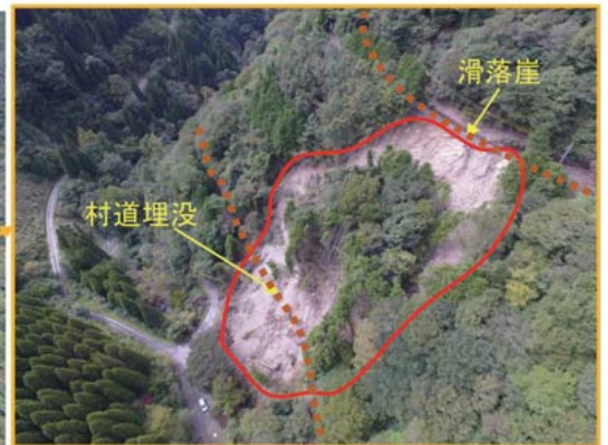
村道白蔵線(下梶原)地すべり現場 (撮影日平成29年10月)
